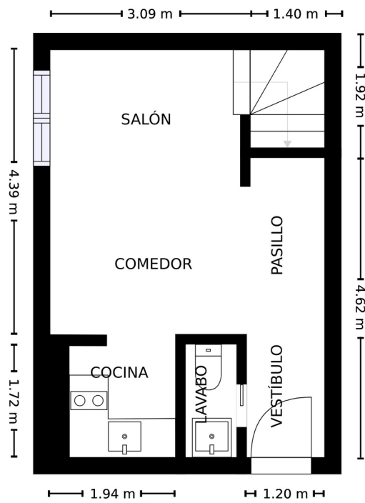
1. PLANTA
