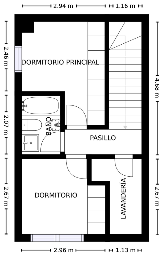
2. PLANTA
